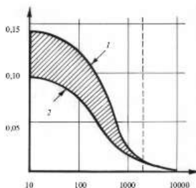
Рис. 1. Влияние модификатора трения на коэффициент трения:
