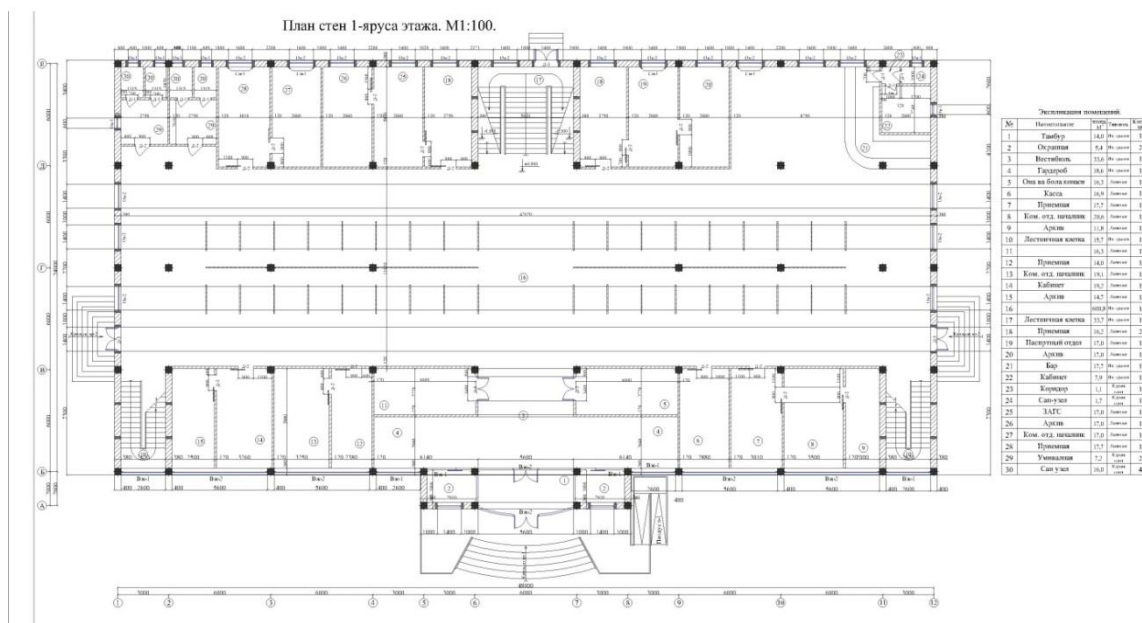
2-расм. Хоразм вилояти Урганч шаҳар марказида жойлашган Давлат хизматлари агентлиги маркази биносининг биринчи қават тарх лойиҳаси
