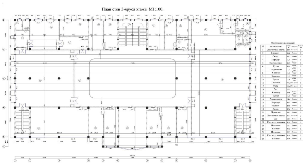
4-расм. Хоразм вилояти Урганч шаҳар марказида жойлашган Давлат хизматлари агентлиги маркази биносининг учинчи қават тархи.
