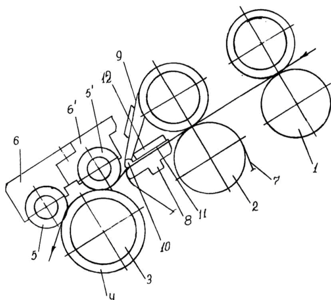
Рис. 1. Двух ремешковый вытяжной прибор. 1-питающая пара; 2,3-вытяжные пары; 4-нижний цилиндр; 5, 5'-ролики; 6, 6'-седелки; 7, 9-ремешки; 8-планки; 10-направитель; 11-пластина; 12-постоянный магнит.
